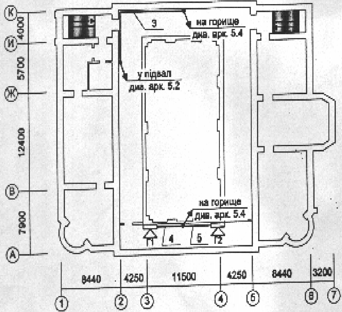
План Балкону на відм. +10.270
